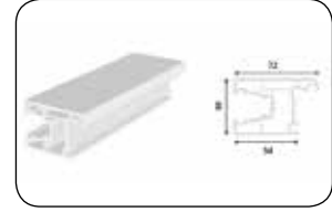
YENİ SÜRME KANAT PROFİLİ
