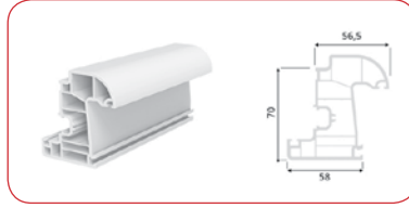
OVAL DAMLALIKLI KANAT PROFİLİ
