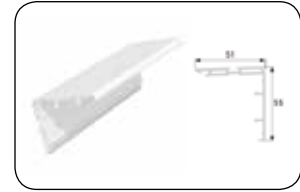
CONTALI KAPI KANAT KAPAMA PROFİLİ
